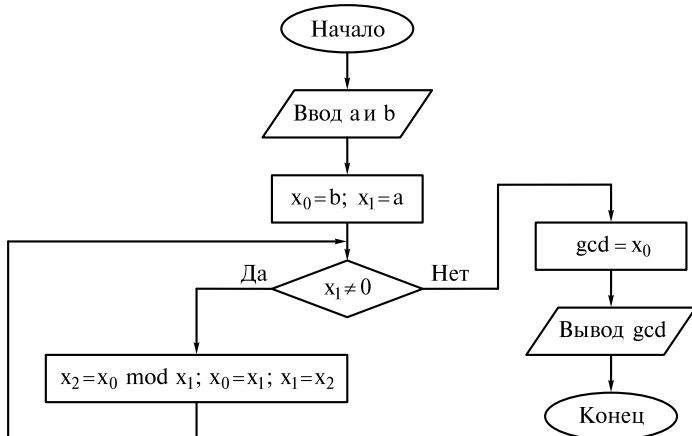
Рис. 1.1. Блок-схема алгоритма для нахождения наибольшего делителя
